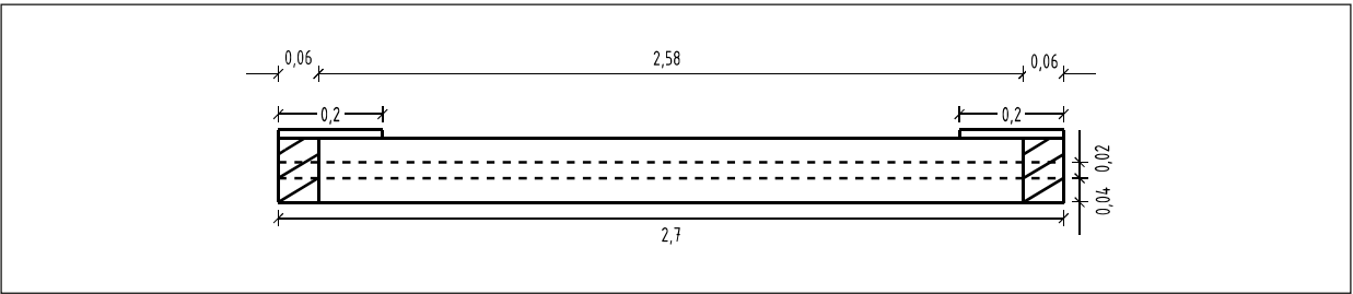
Ansicht Breitseite
