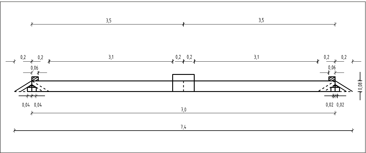
Ansicht Längsseite
